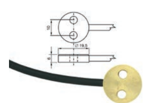
Pt1000TG7/E (-30°C až +200°C)
