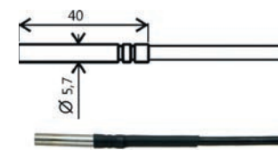
Pt1000TG8/E (-80°C až +200°C)
